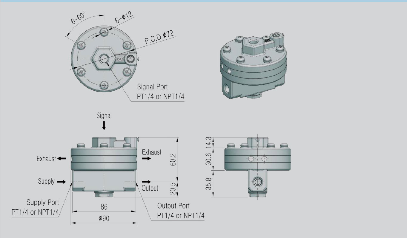
Размеры клапана
