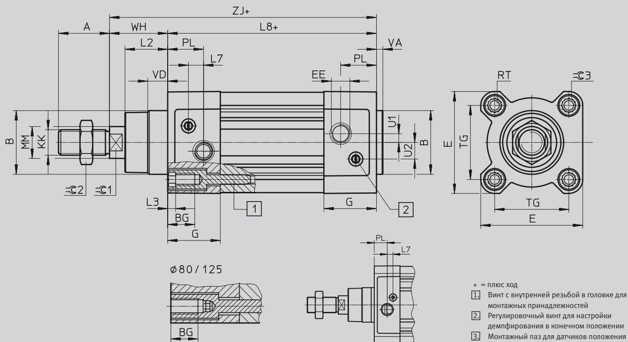
Стандартный пневмоцилиндр DSBC по ISO 15552
