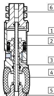
DHEB-...-U
