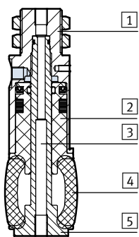
DHEB-...-D
