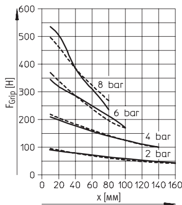
HGP-35-A-B
