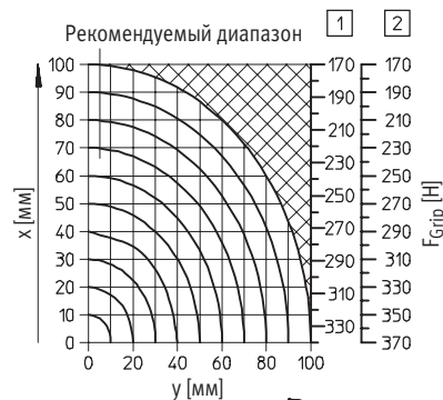
HGP-35-A-B
