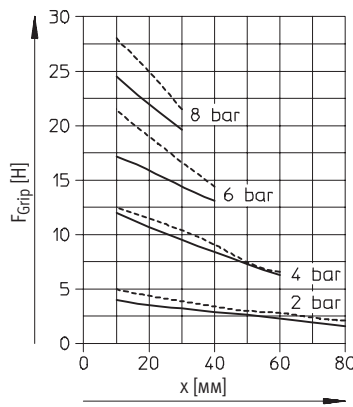
HGP-10-A-B
